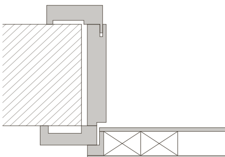
Umfassungszarge: Zarge für gefälzte Türen
