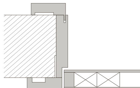
Zarge für stumpfe Türen
